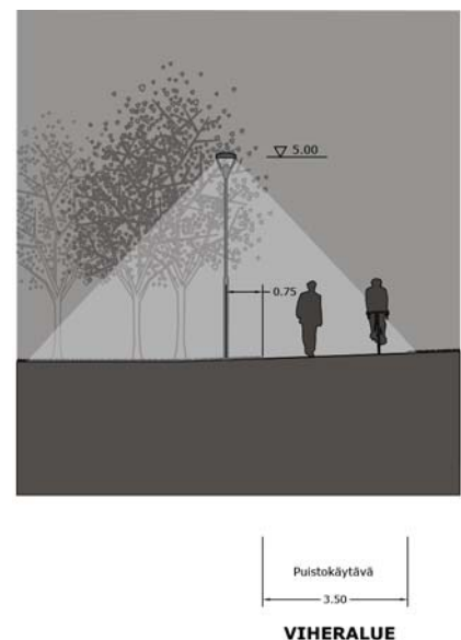
Kuva 27. Puistokäytävän tyyppipoikkileikkaus.
