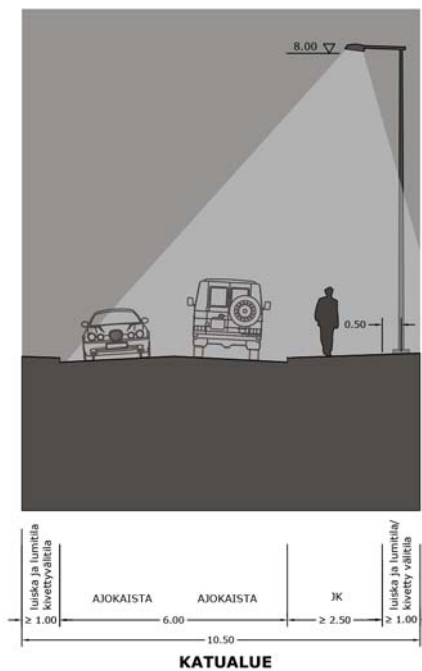
Kuva 18. Tonttikadun tyyppipoikkileikkaus työpaikka-alueella. (Tyyppipoikkileikkauksen pohja: Vantaan katutila -raportti 2010)
