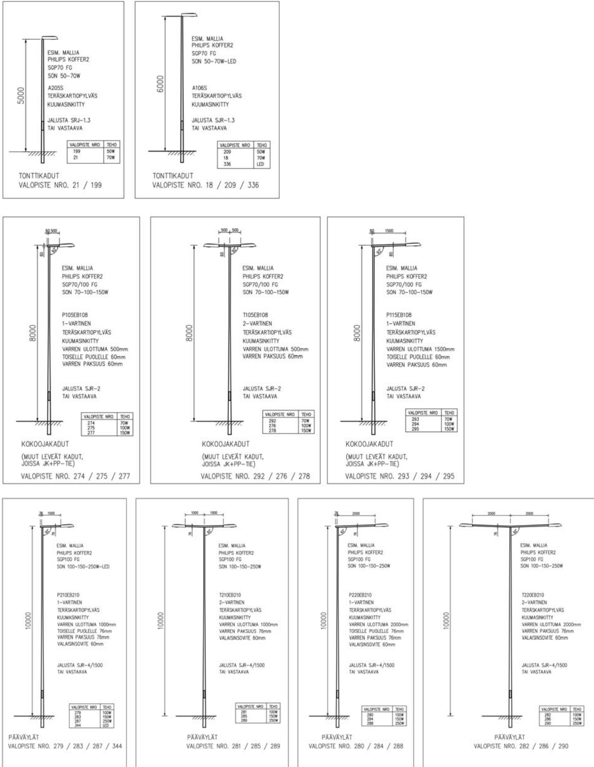
Kuva 51. Vantaalla käytettävä valaisinpylväsmallisto. (Kuva Vantaan katutila, mitoitus ja laatu 2010)
