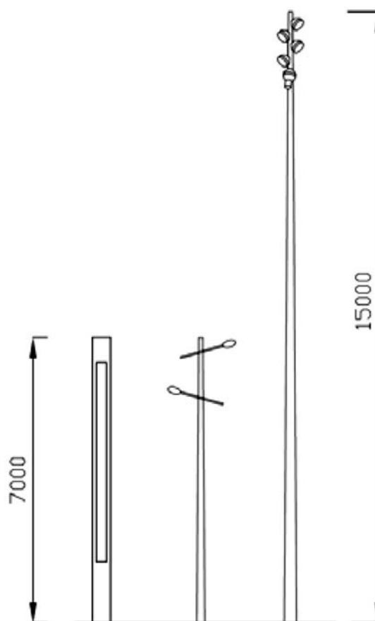
Kuva 19. Tikkuraitilla käytettäväksi ehdotettuja valaisimia. (Ote Tikkurilan keskustan yleissuunnitelmaraportista Ramboll 2009).
